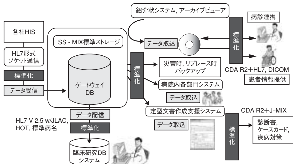
図1 SS-MIX標準ストレージを利用したデータの流れ
